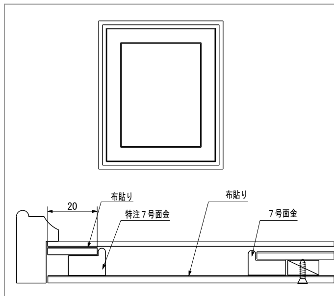
商品図面
