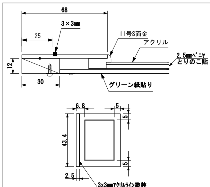
商品図面
