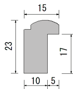
外枠断面図
