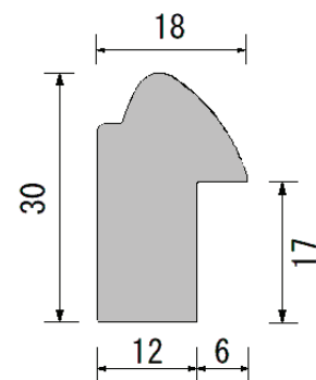
外枠断面図
