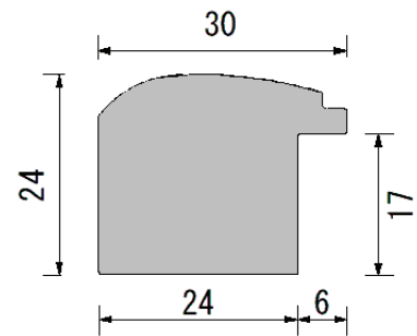
外枠断面図
