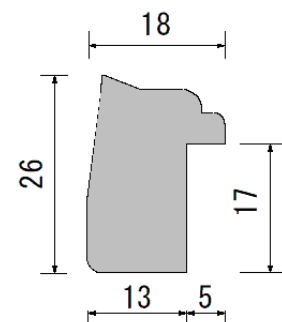
外枠断面図
