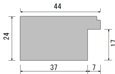
外枠断面図
