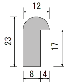
外枠断面図
