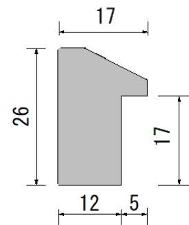
外枠断面図
