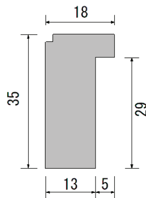
外枠断面図
