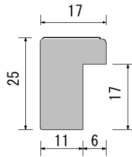
外枠断面図
