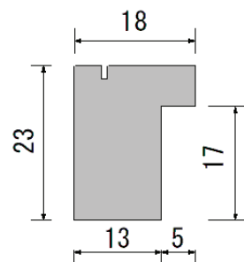
外枠断面図
