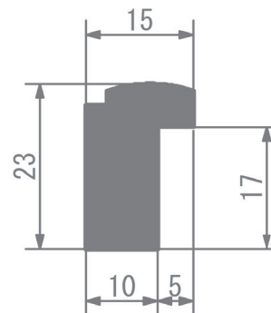
外枠断面図
