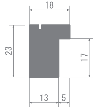
外枠断面図
