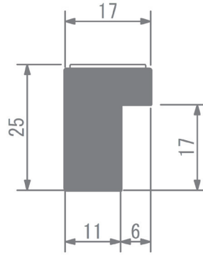
外枠断面図
