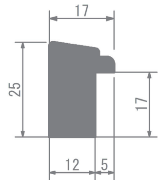
外枠断面図
