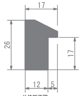
外枠断面図
