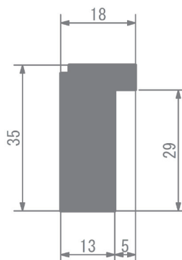
外枠断面図
