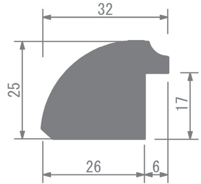
外枠断面図
