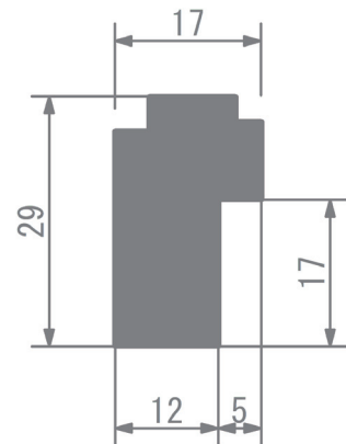
外枠断面図
