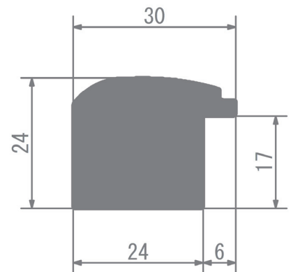
外枠断面図
