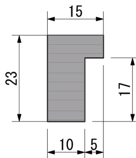
外枠断面図
