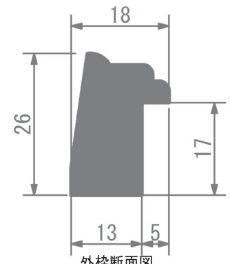
外枠断面図
