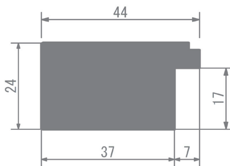
外枠断面図
