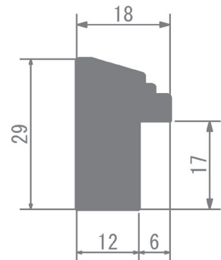
外枠断面図
